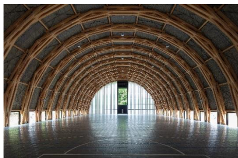
奈良の木を利用した移動式仮設体育館
